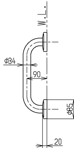
取付座詳細(1:2)
